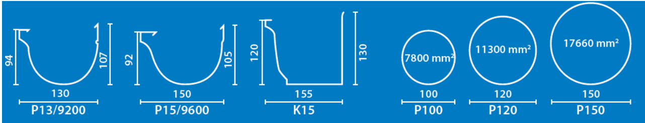
Bild 1. Tvärsnittsområden
