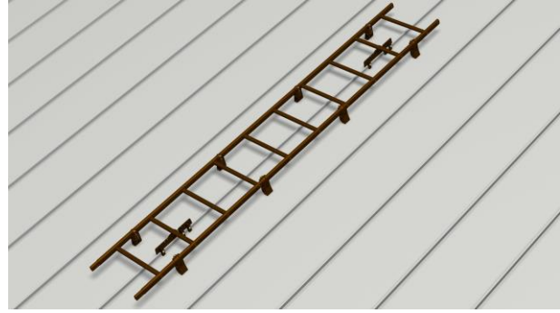
Kuva 4. Lukkosaumakatto
