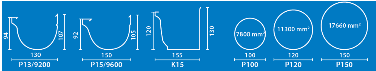
Kuva 1. Läpileikkauspinta-alat
