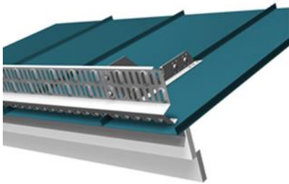
Kuva 1. PLE/VARMA 120 konesaumakatonle
