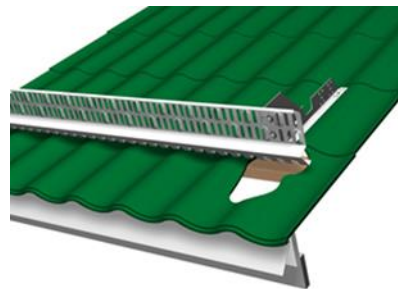
Kuva 2. PLE/VARMA 120 tiilikatonle
