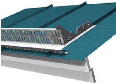
Kuva 3. PLE/VARMA 120 Classic-katonle
